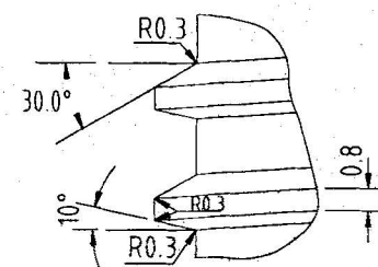
Einzelheit Y - detail Y -
