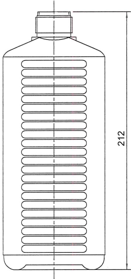
Seitenansicht von Links Side view left
